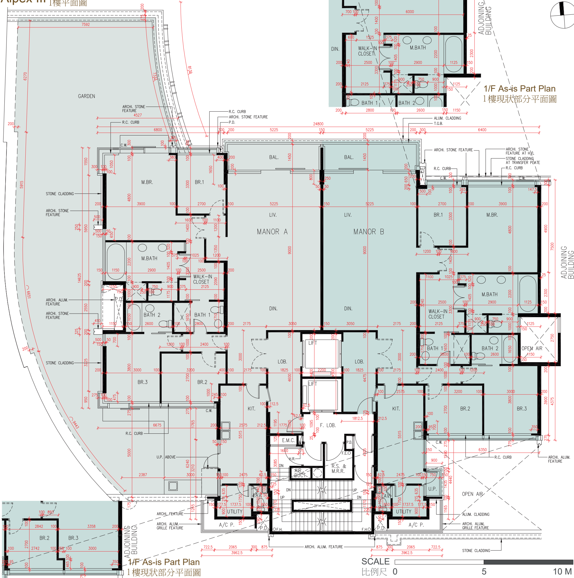
Alpex III 1/F Plan 1樓平面圖
