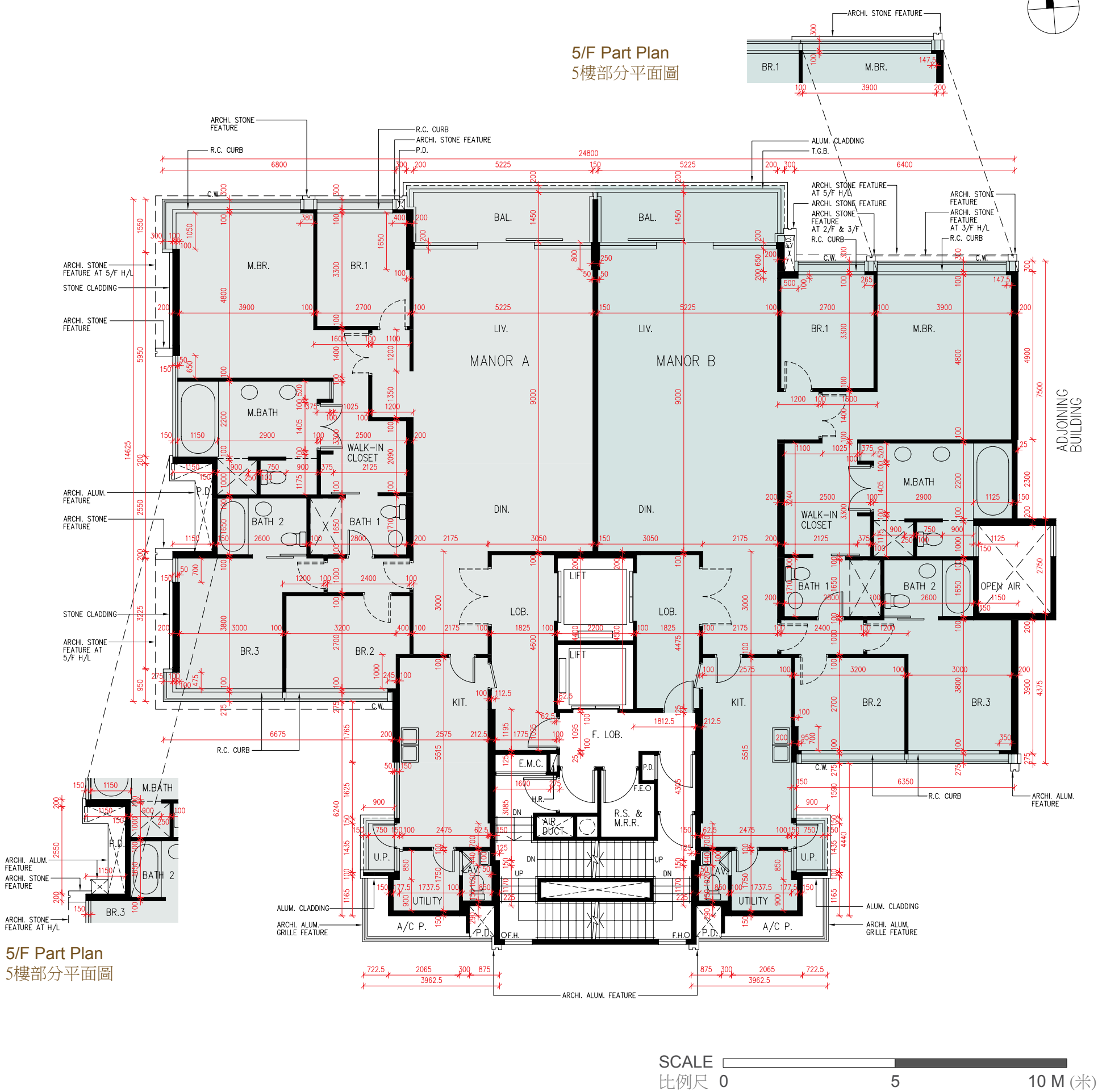
Alpex III 2/F, 3/F & 5/F Plan 2樓、3樓及5樓平面圖
