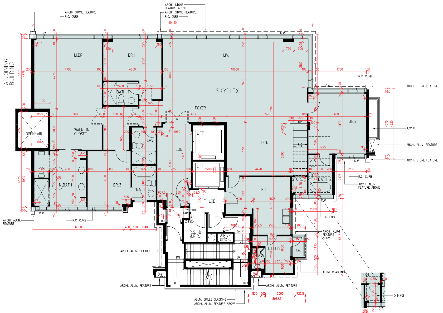
7/F As-is Part Plan 7樓現狀部分平面圖
