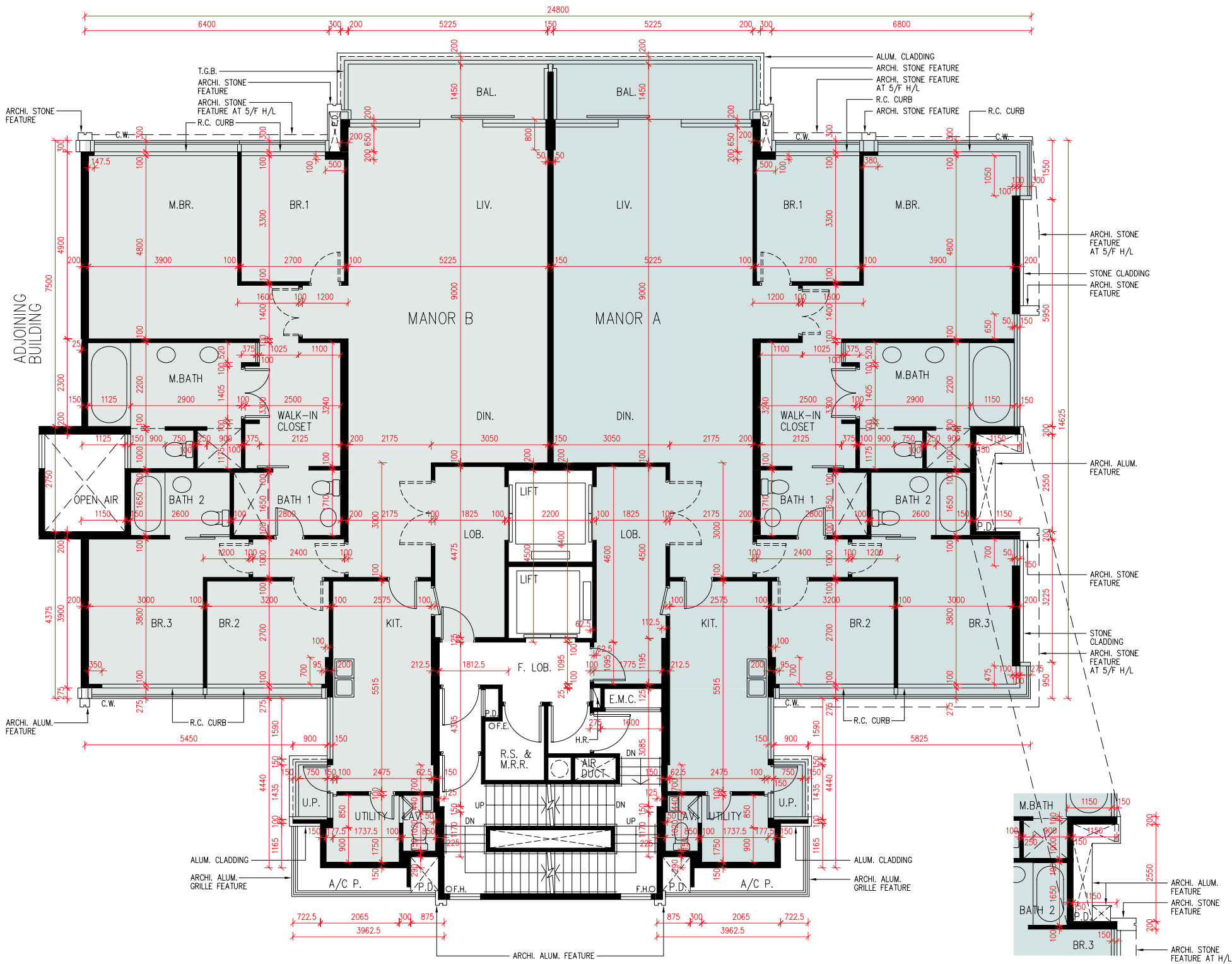
5/F Part Plan 5樓部分平面圖
